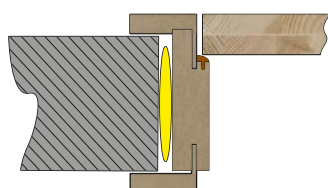
ościeżnica Standard 80 szerokość opaski 80 mm
