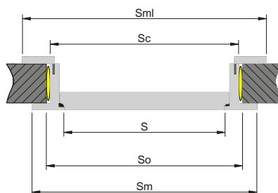
Przekrój poziomy drzwi
