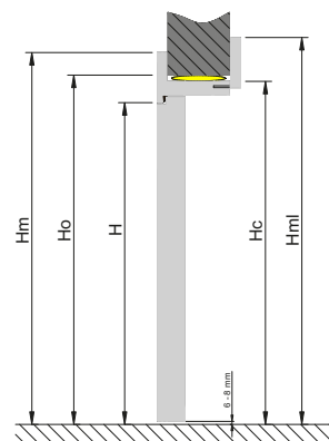
Przekrój pionowy drzwi
