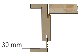
przekrój przez ościeżnicę zakres regulacji 30 mm
